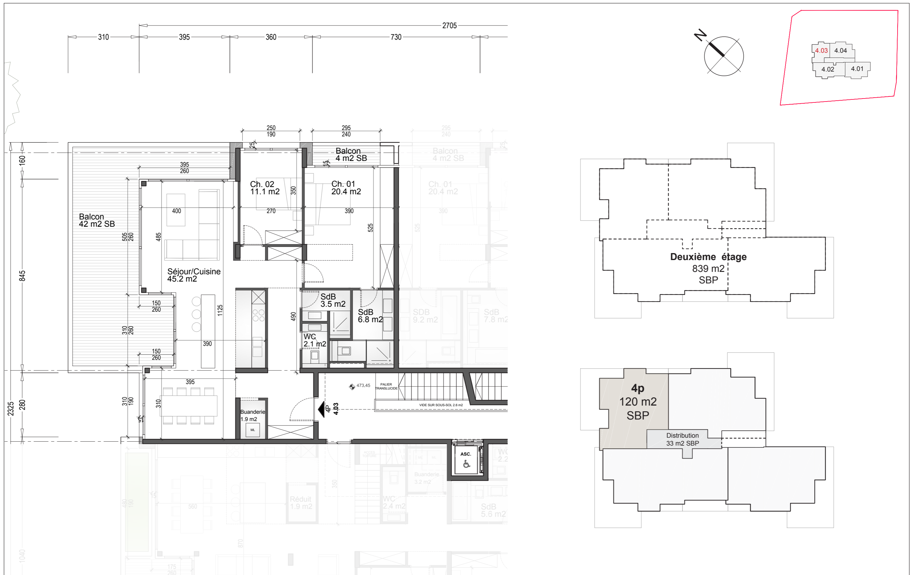
Plan typologie, Deuxième étage , appartement 4.03 1:100
