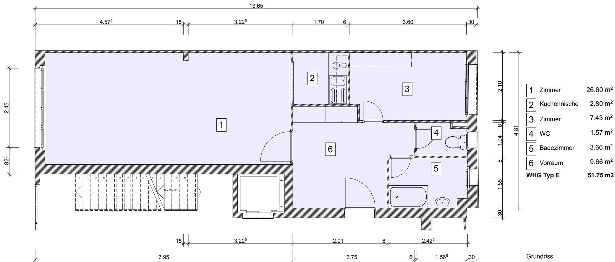
Wohnung Typ E 51.75 m 2
