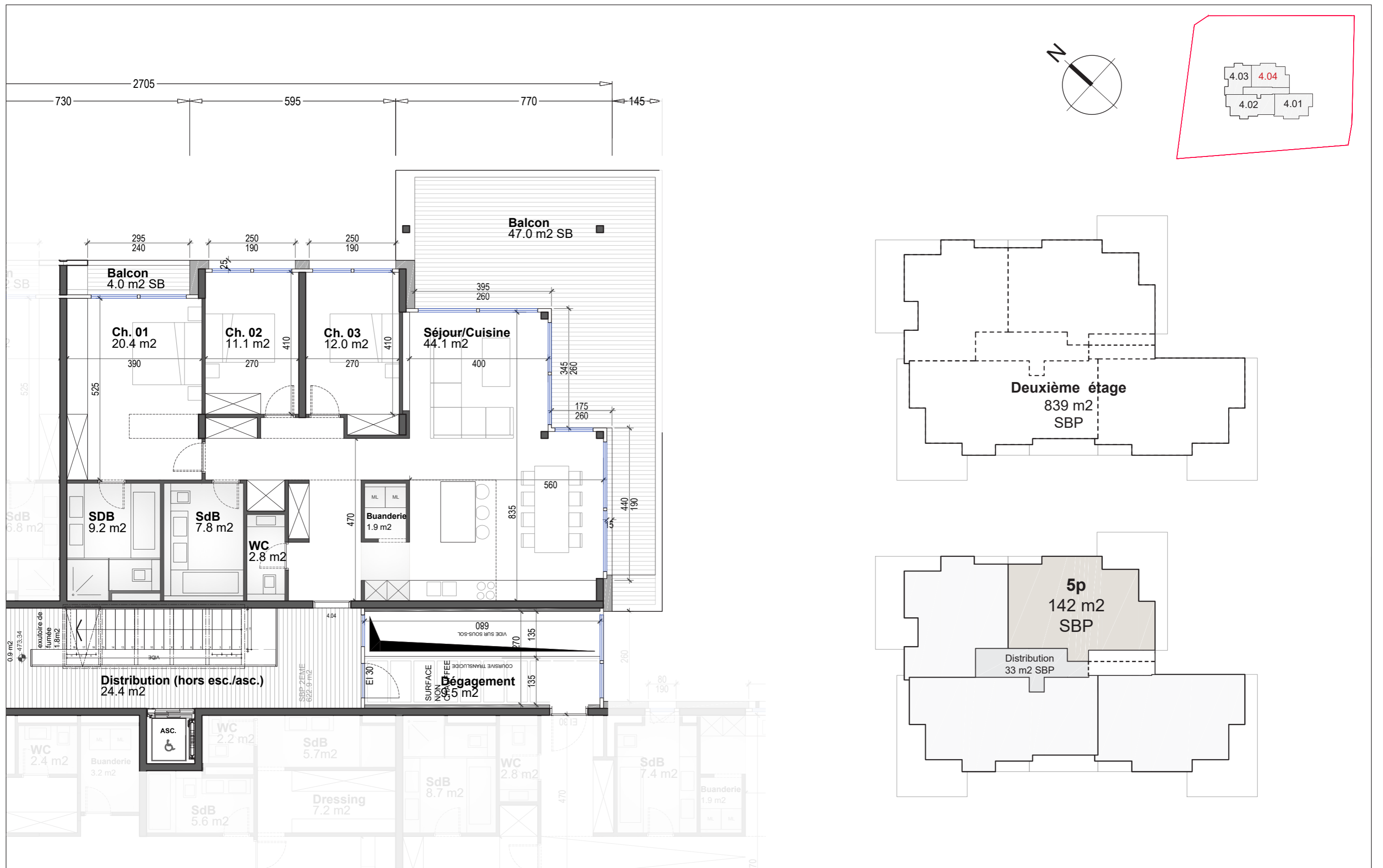
Plan typologie, Deuxième étage , appartement 4.04 1:100
